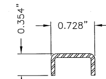
9 SASH REINFORCEMENT VEKA #RFSH45 SOM
