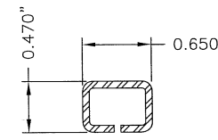
10 LOCK RAIL REINF. VEKA #RFSH46 SOM
